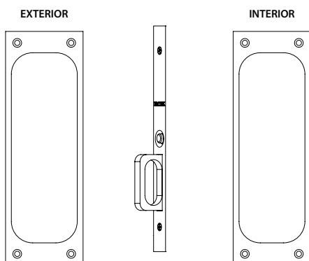
Passage Door Mortise Lock
